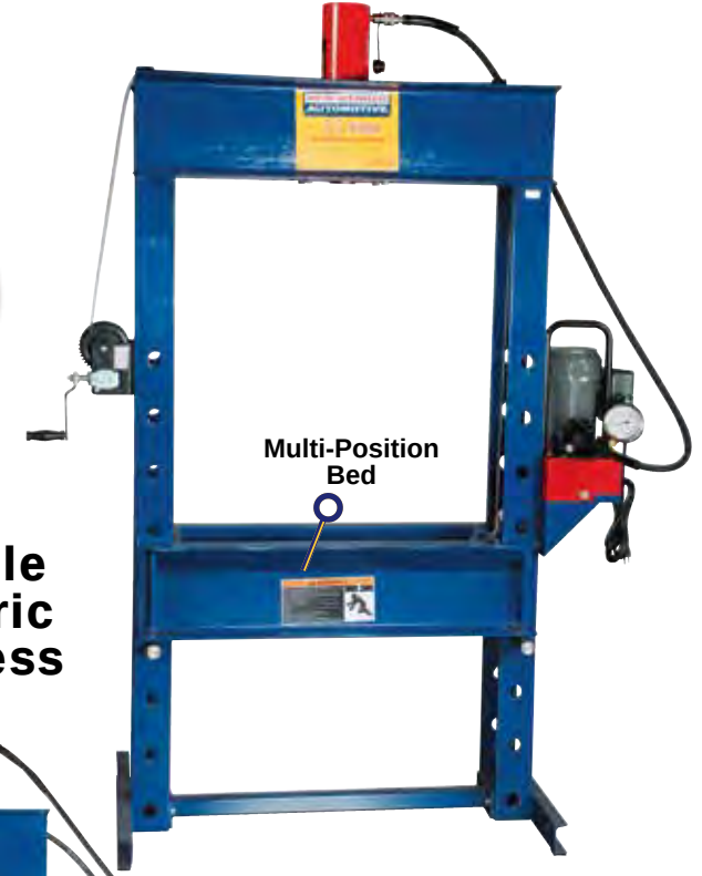
55 Ton Electric Hyd Shop Press
